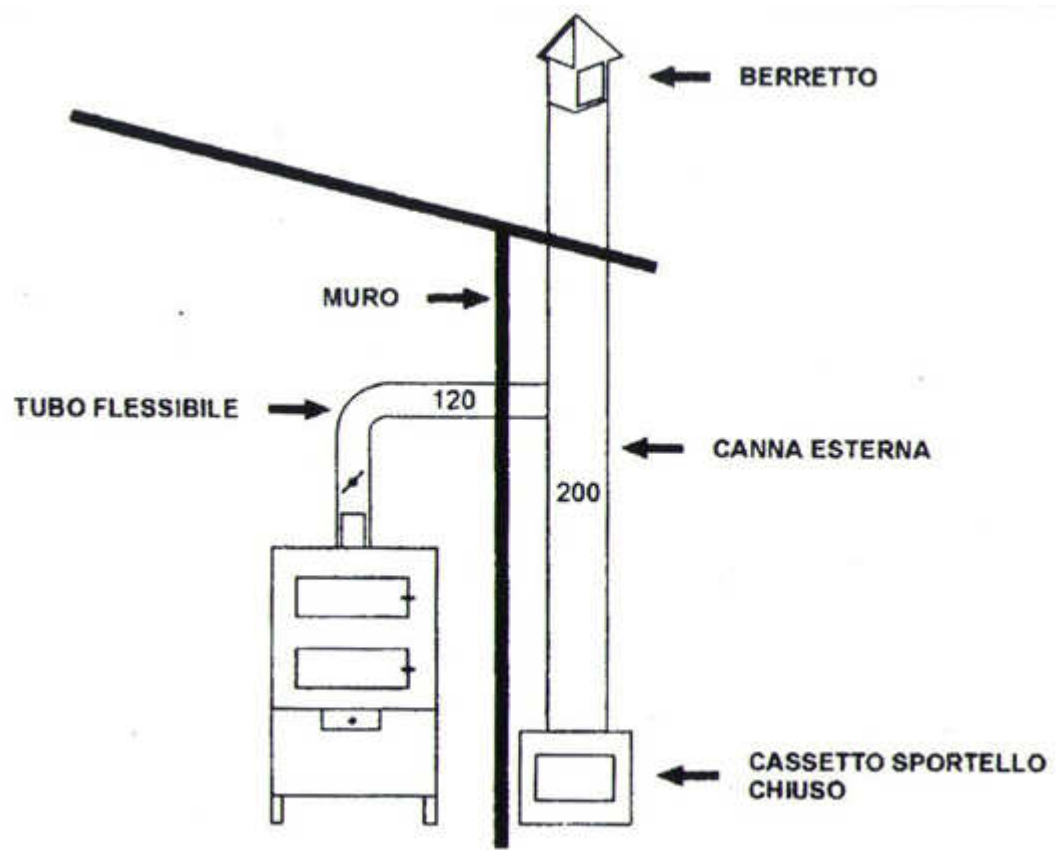
SISTEMA CORRETTO DELLA CANNA FUMARIA
