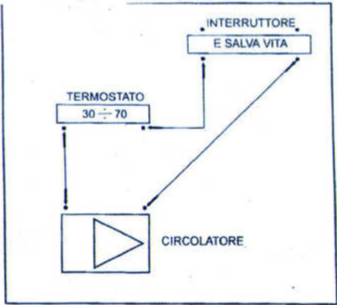
SCHEMA ELETTRICO
