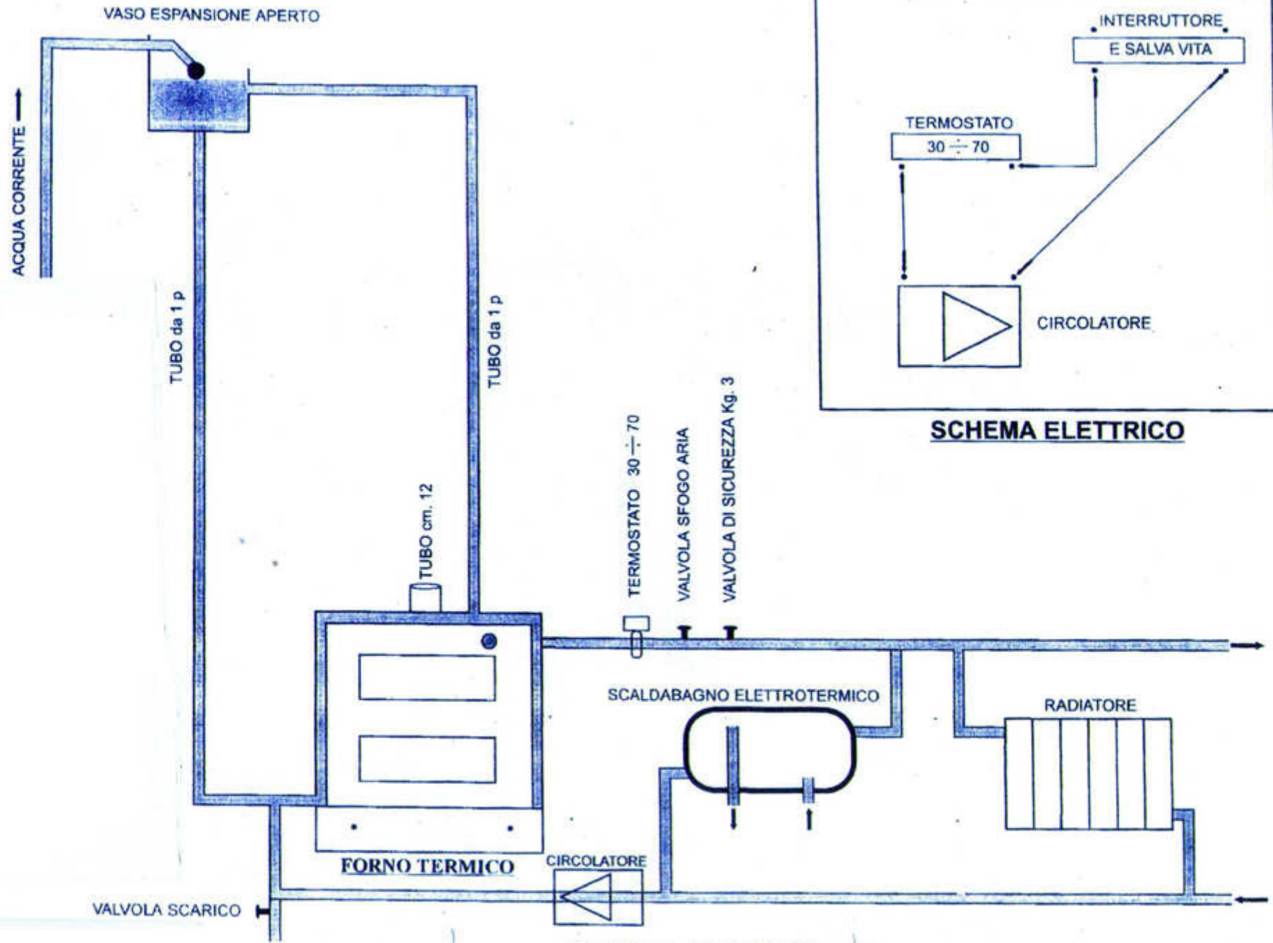
SCHEMA IDRAULICO
